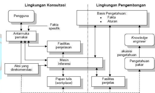
Gambar 1. Struktur Sistem Pakar
