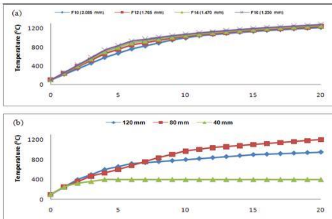
Gambar .3 profil Suhu di dalam reactor
