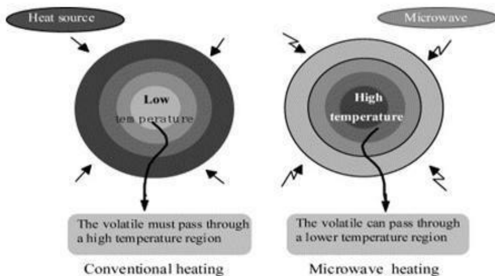
Gambar 1. Perbandingan pemanasan konvensional dengan pemanasan microwave
