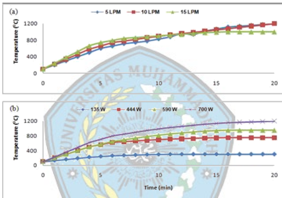
Gambar 4. profil suhu di dalam reactor
